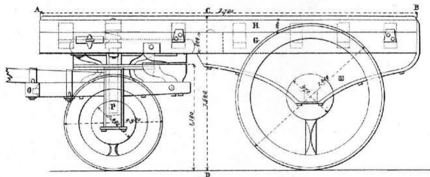
Fig.1 Elevation
